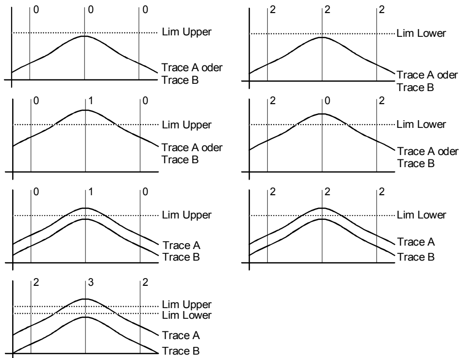
Bild 2-38 Kode der Limitverletzungen anhand einiger Beispiele
