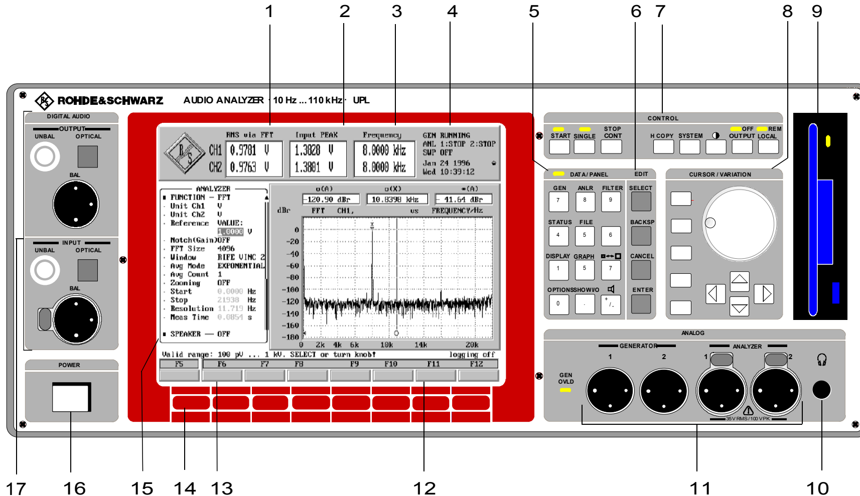
Bild 2-1 Frontansicht
