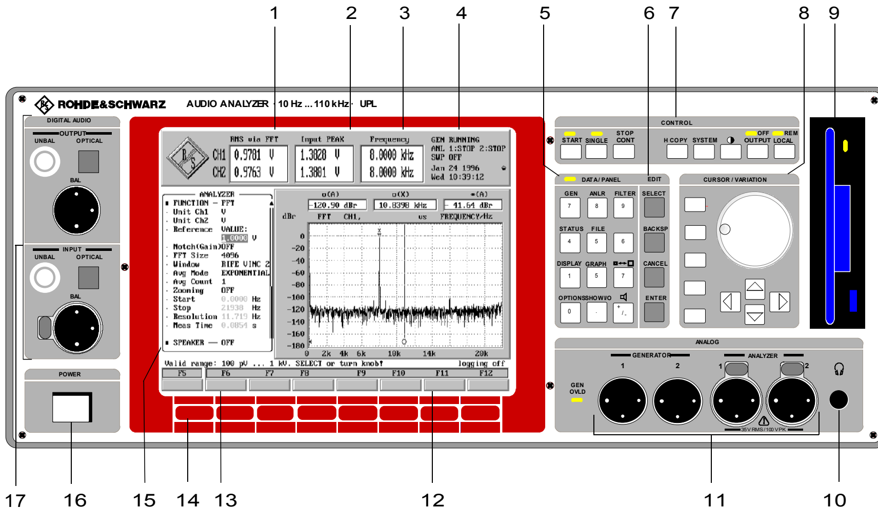
Bild 2-1 Frontansicht
